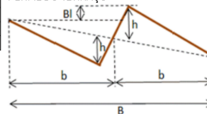
PERFIL DO TERRAÇO
