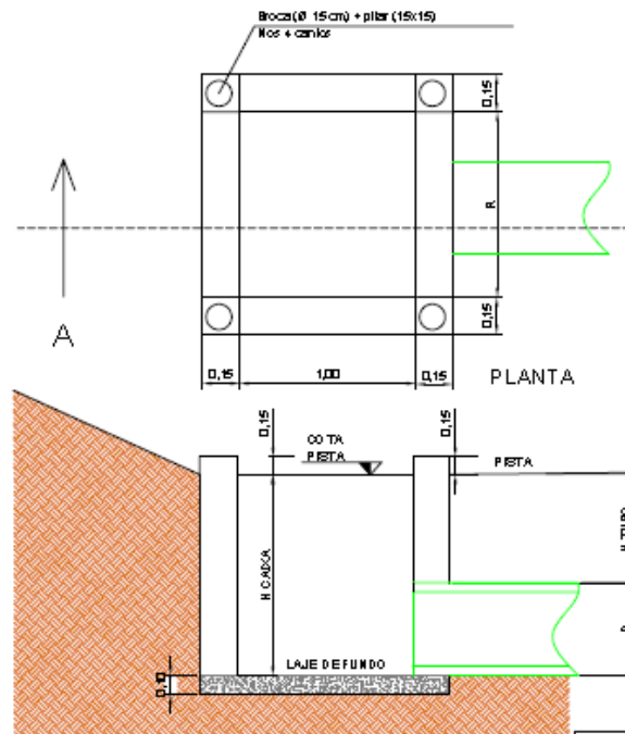
CORTE AA DETALHE DE CAIXA DE CAPTAÇÃO
