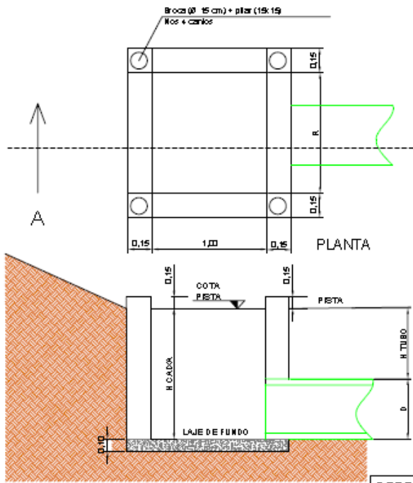
CORTE AA DETALHE DE CAIXA DE CAPTAÇÃO
