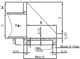
DETALHE DE MURO DE ALA SEM ESCALA
