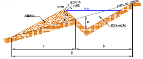
PERFIL DO TERRAÇO SEM ESCALA
