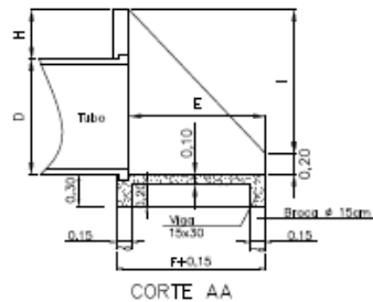
DETALHE DE MURO DE ALA SEM ESCALA
