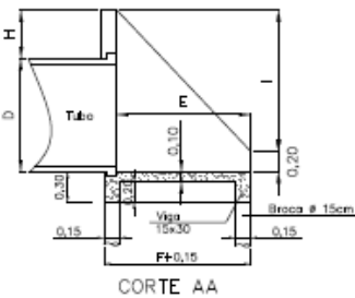
DETALHE DE MURO DE ALA SEM ESCALA
