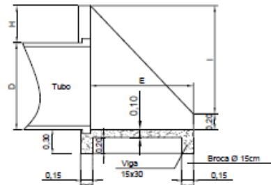
CORTE AA DETALHE DE MURO DE ALA
