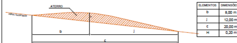
PERFIL DO TERRAÇO
